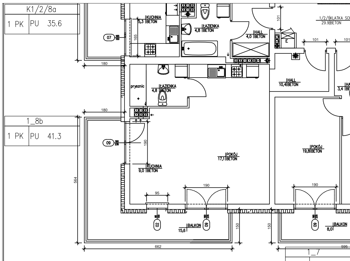
RZUT 2 PIĘTRA:
