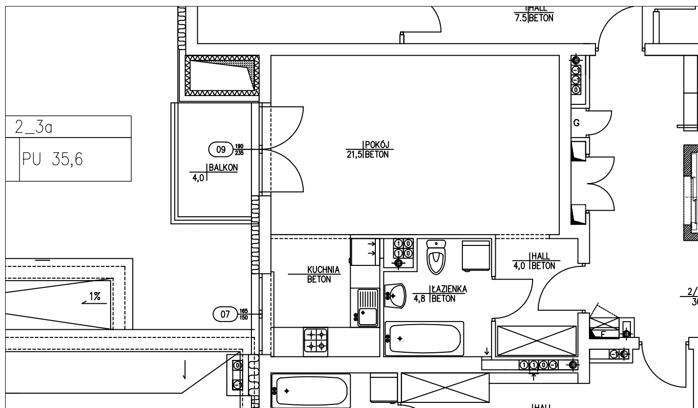
RZUT 1 PIĘTRA:
