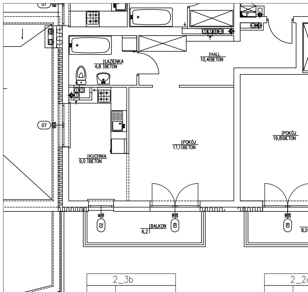
RZUT 1 PIĘTRA:
