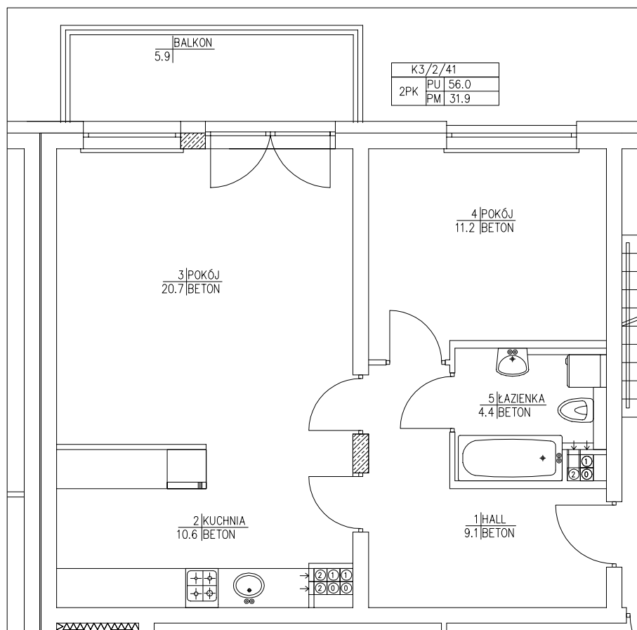
RZUT 2 PIĘTRA:
