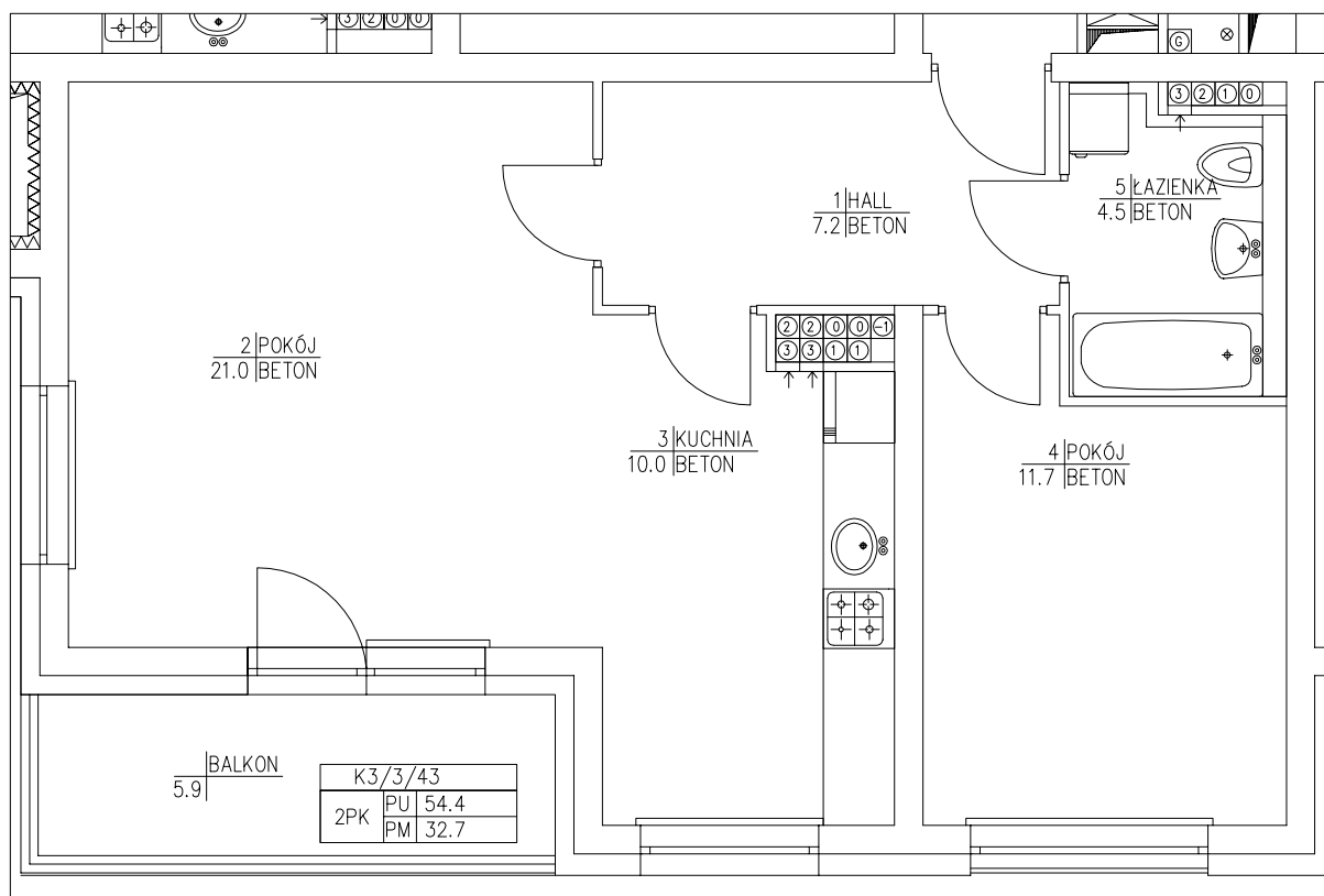
RZUT 3 PIĘTRA:
