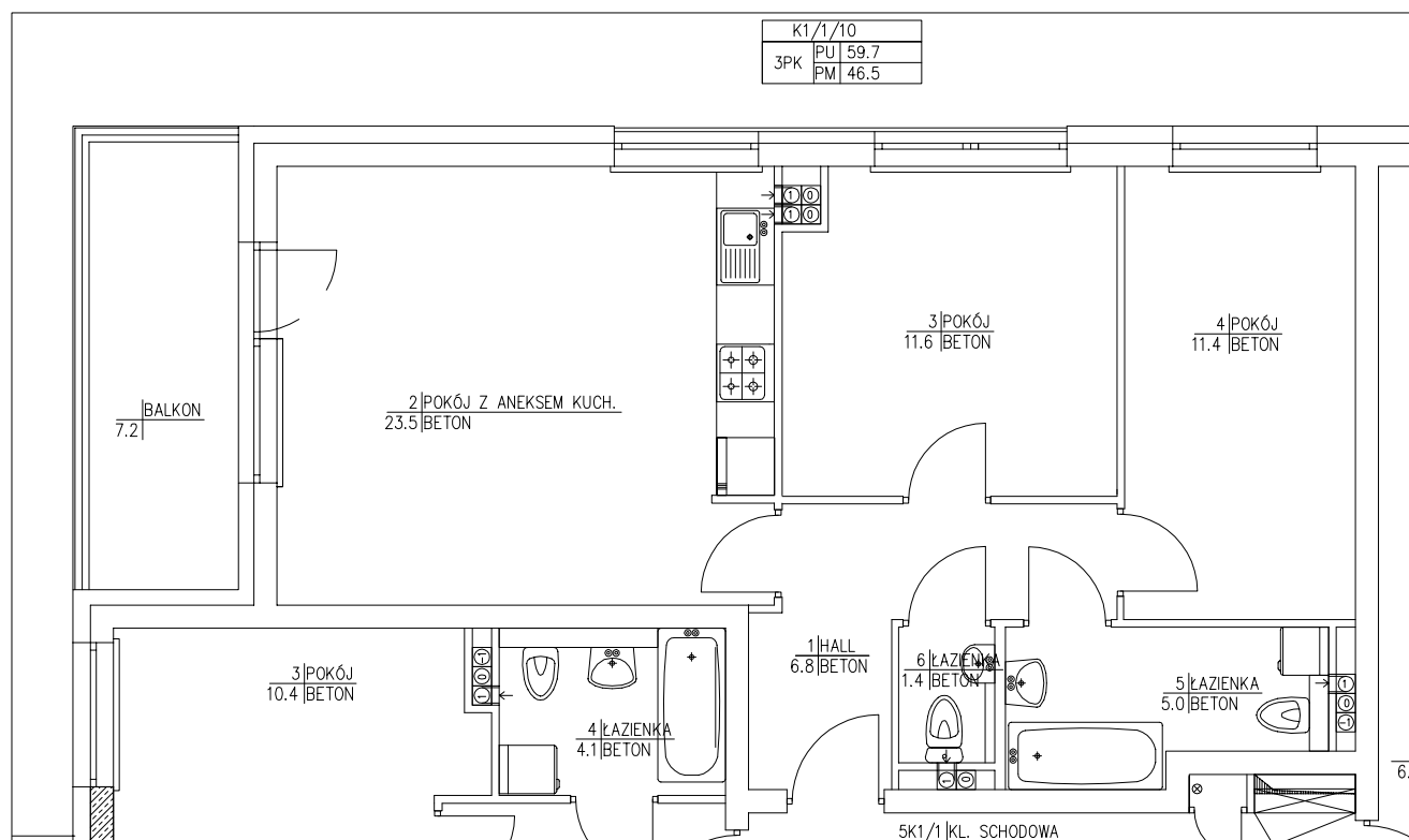
RZUT 1 PIĘTRA:
