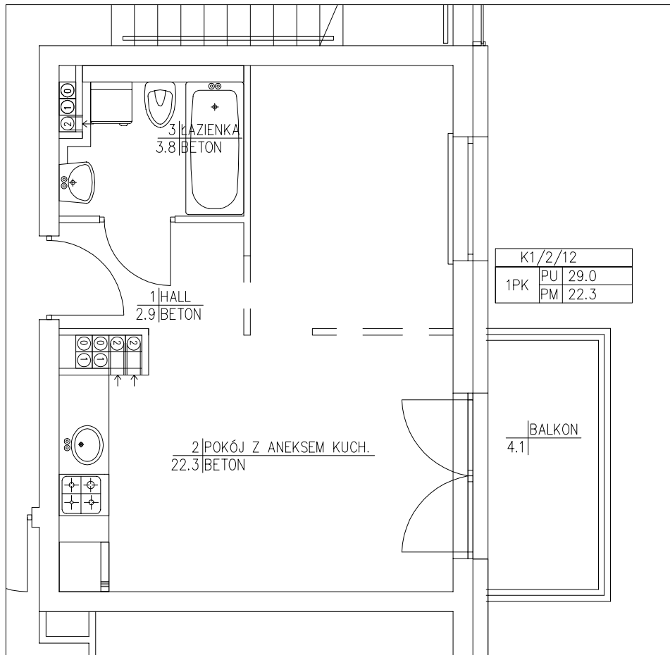
RZUT 2 PIĘTRA:
