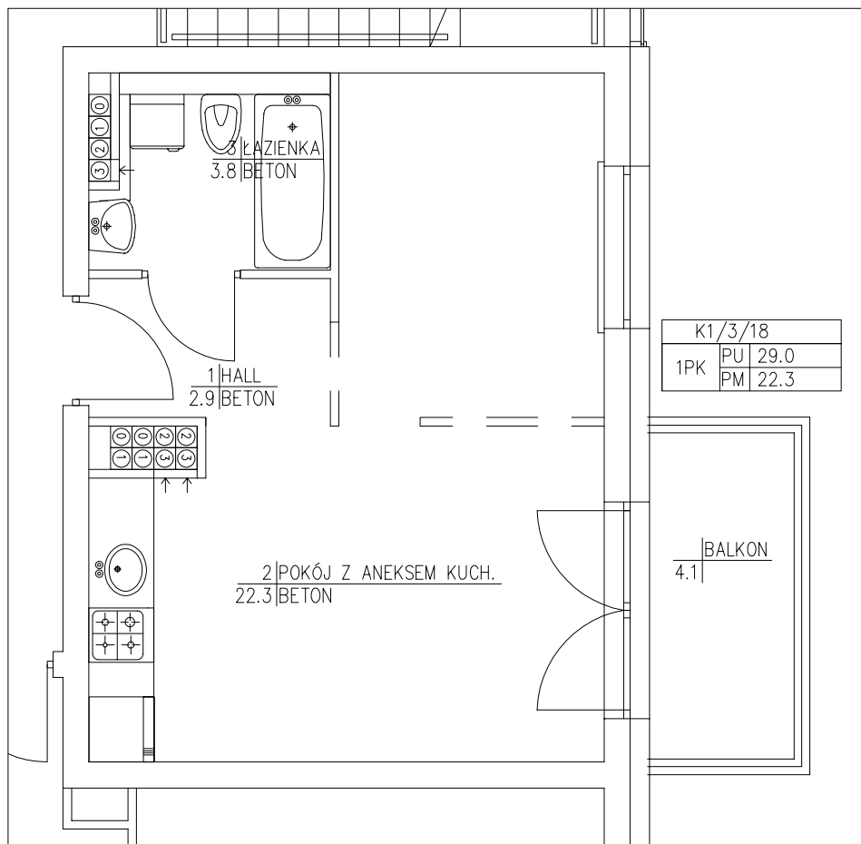
RZUT 3 PIĘTRA:
