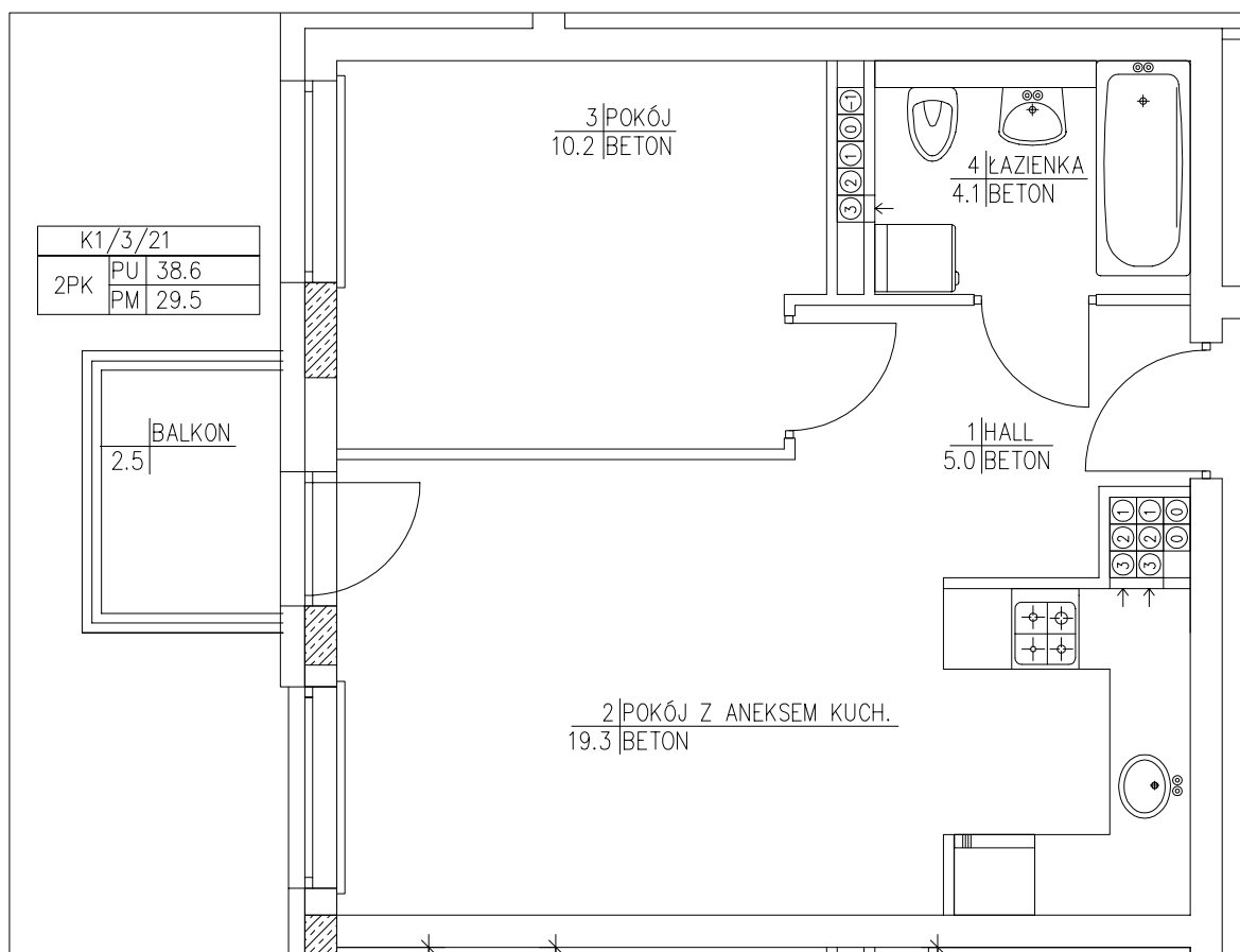
RZUT 3 PIĘTRA:
