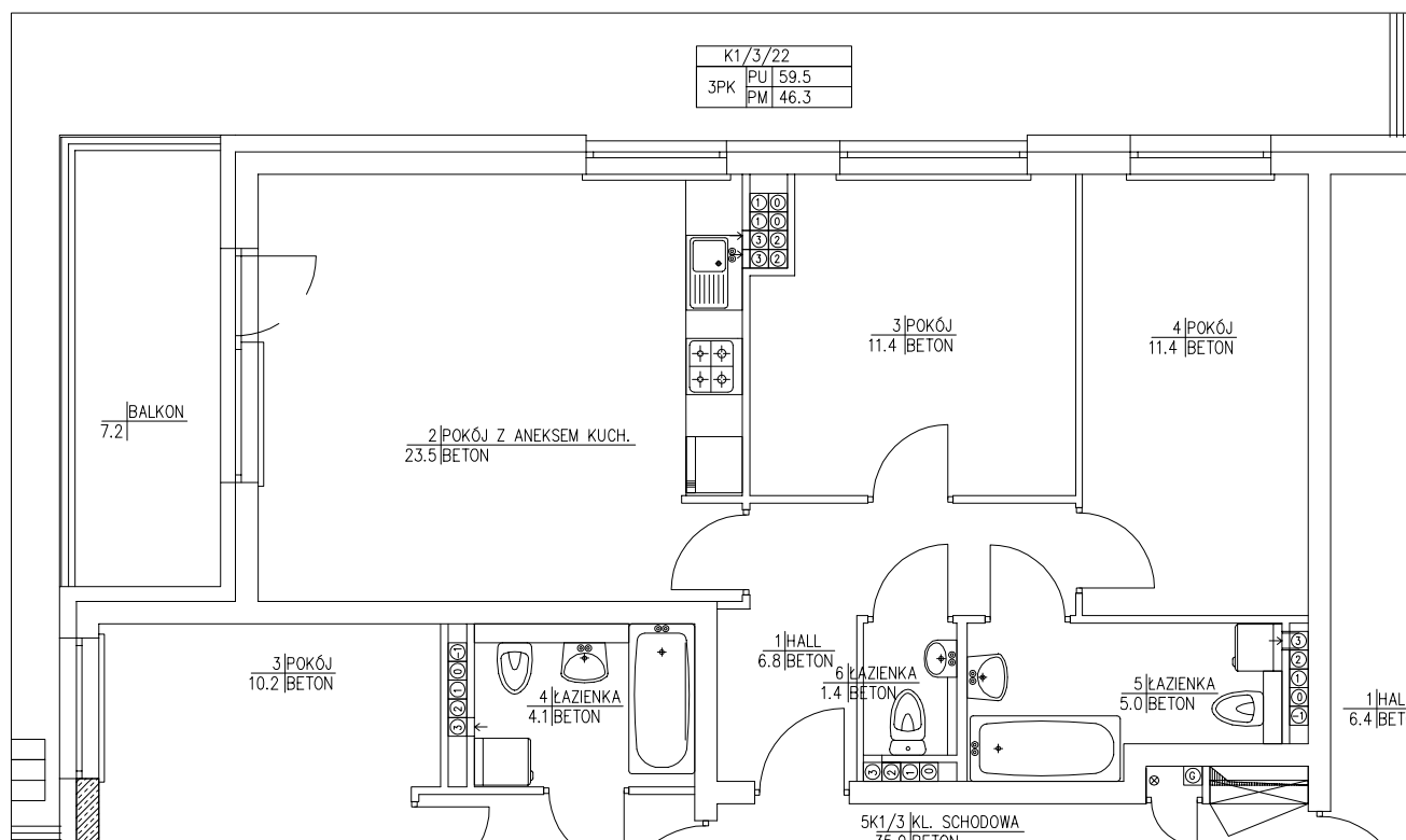
RZUT 3 PIĘTRA:
