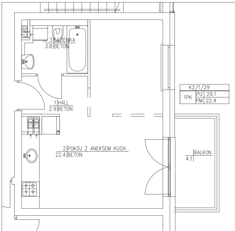
RZUT 1 PIĘTRA:
