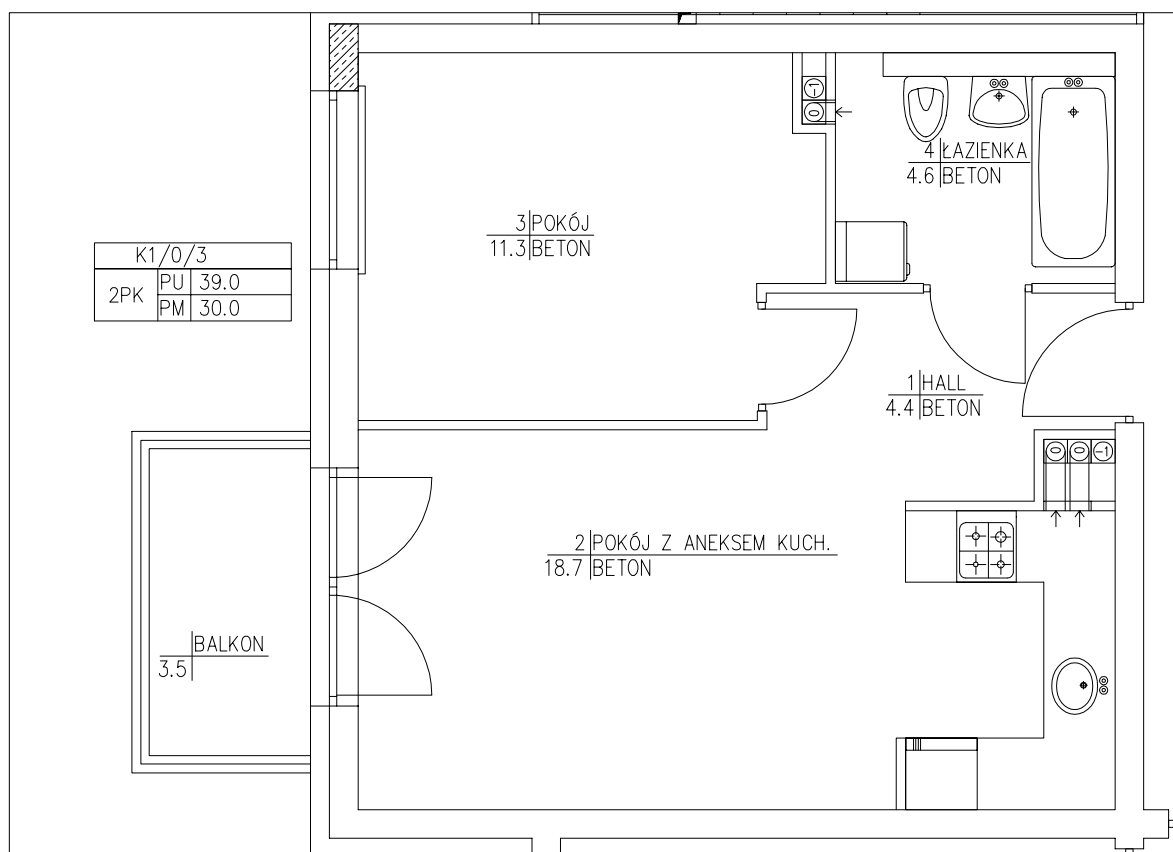
RZUT PARTERU:
