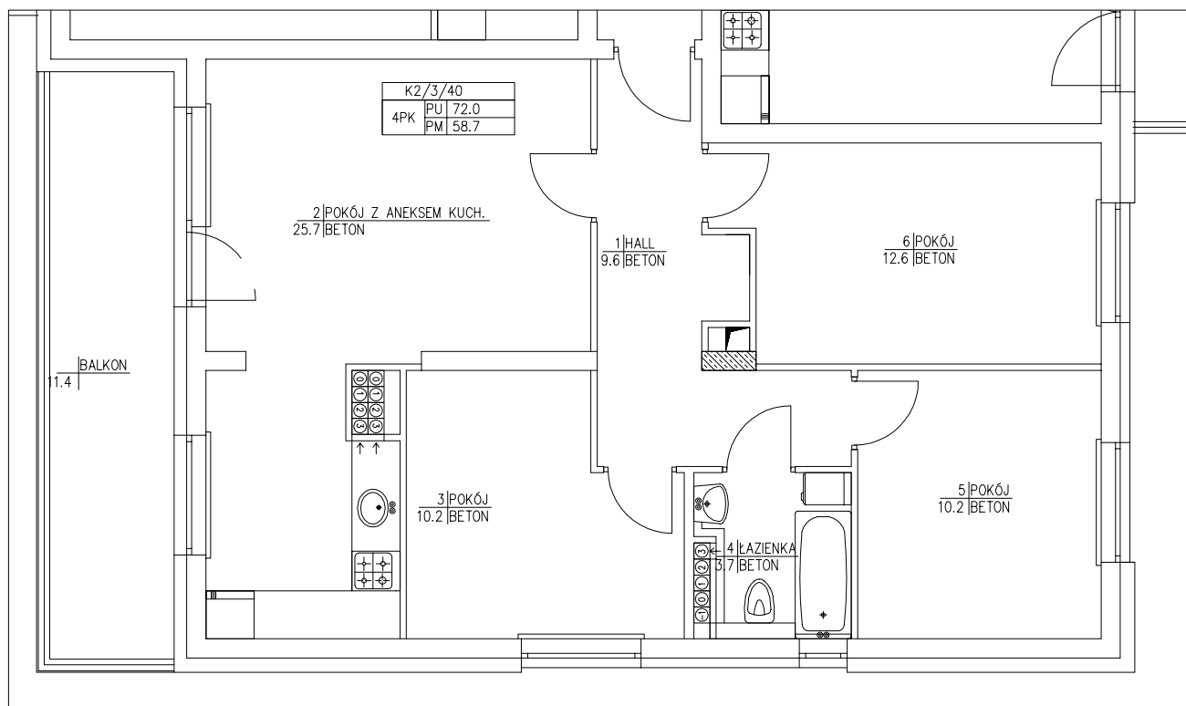
RZUT 3 PIĘTRA:
