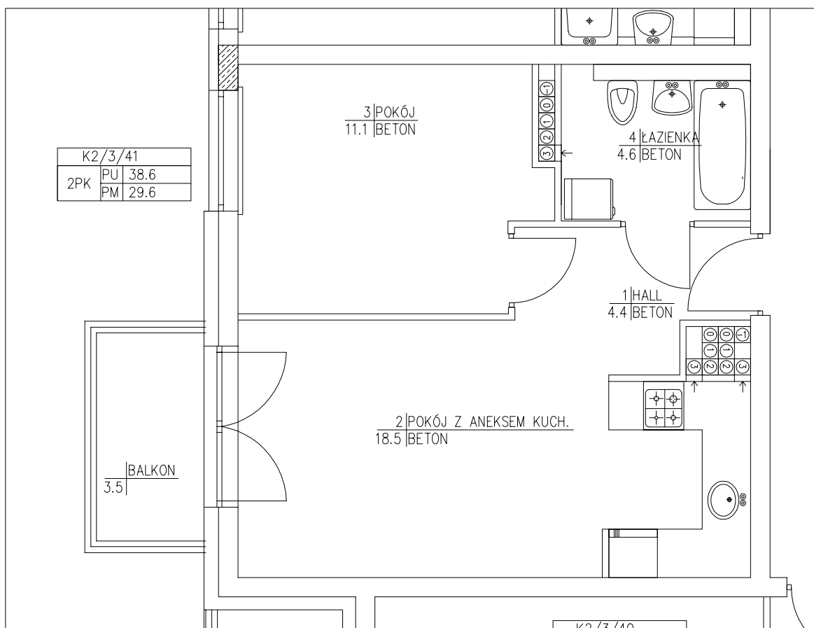
RZUT 3 PIĘTRA:
