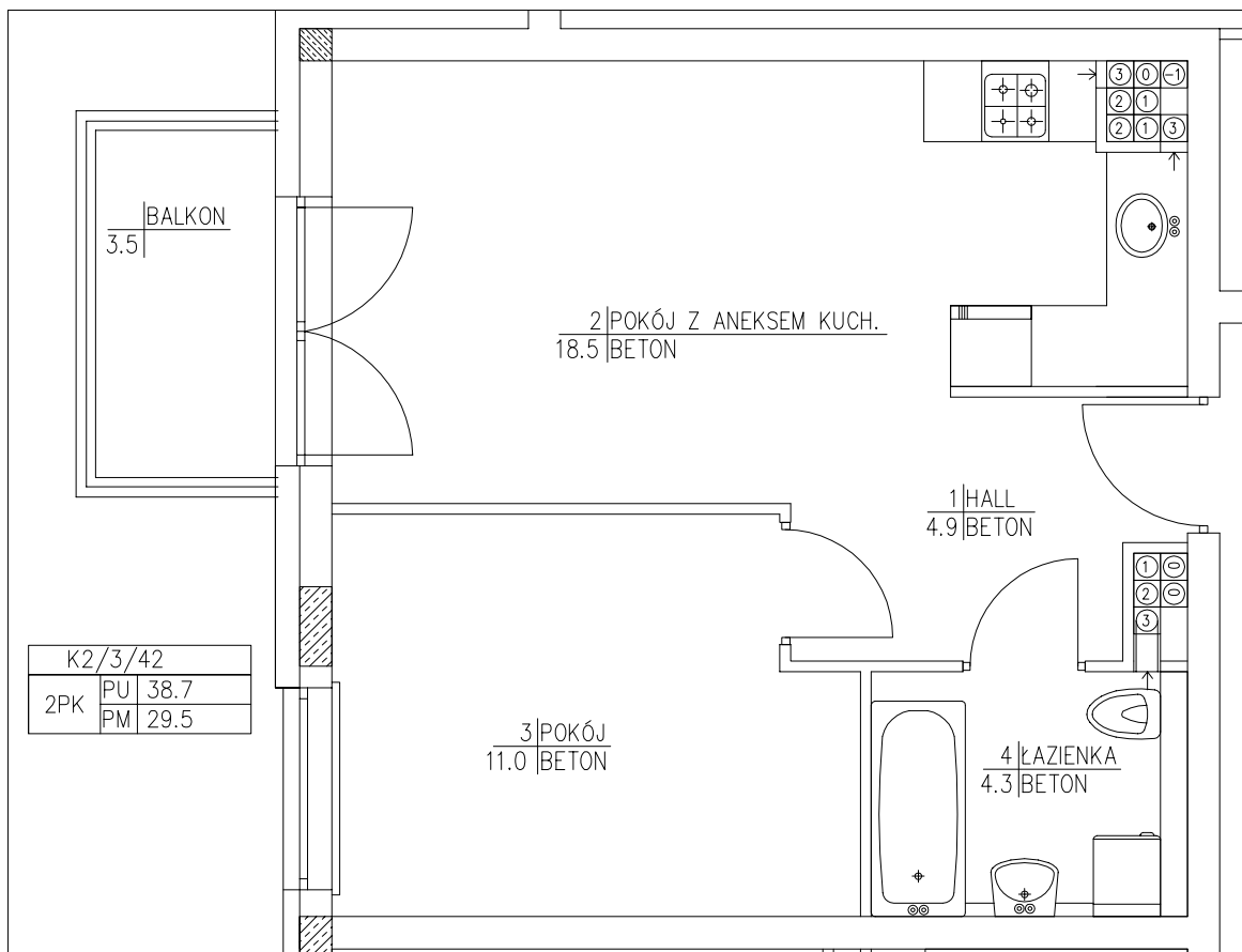
RZUT 3 PIĘTRA:
