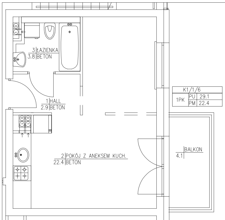
RZUT 1 PIĘTRA:
