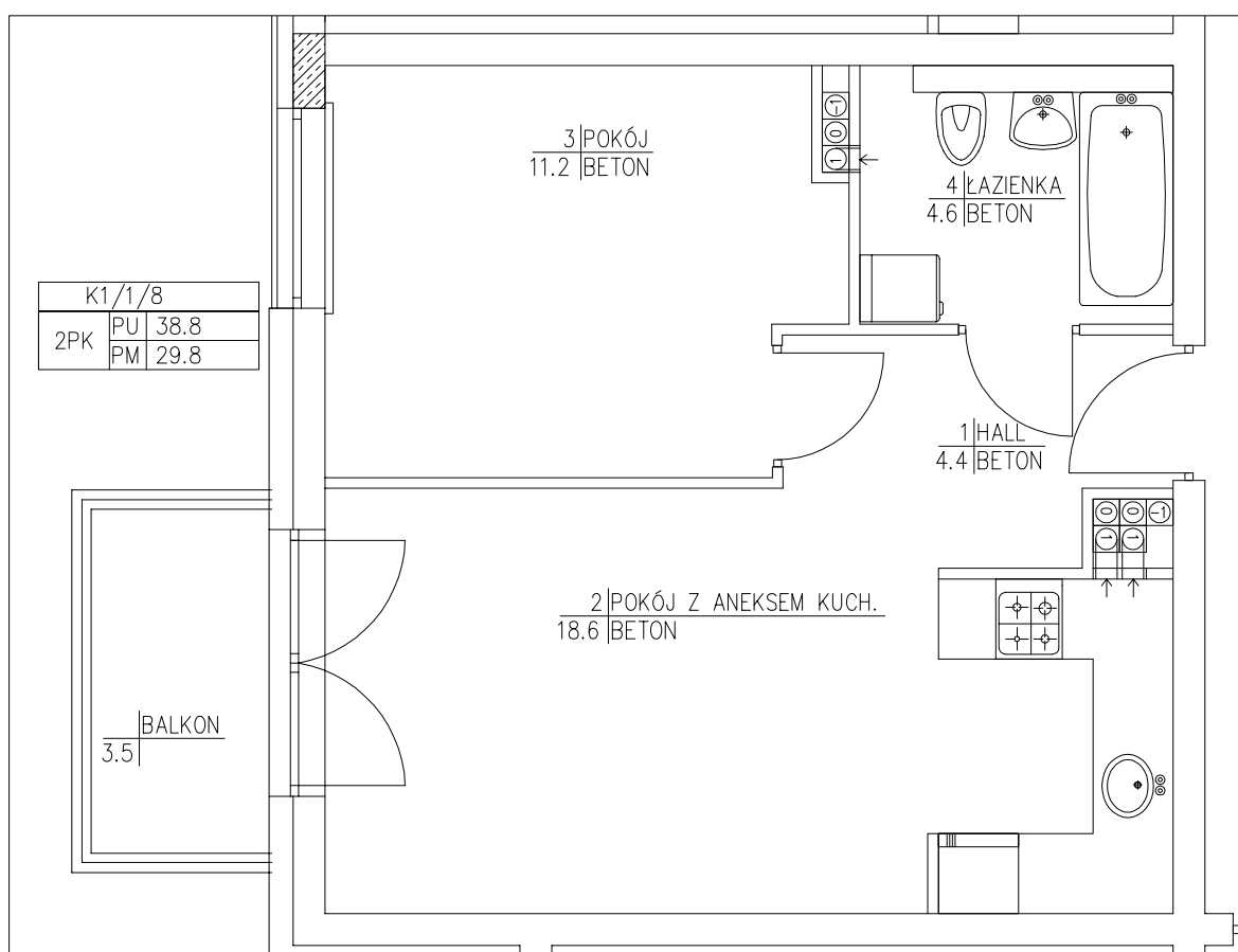
RZUT 1 PIĘTRA:
