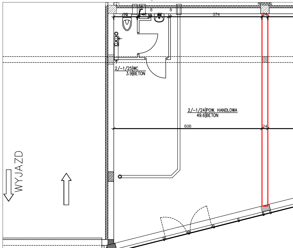
RZUT PARTERU:
