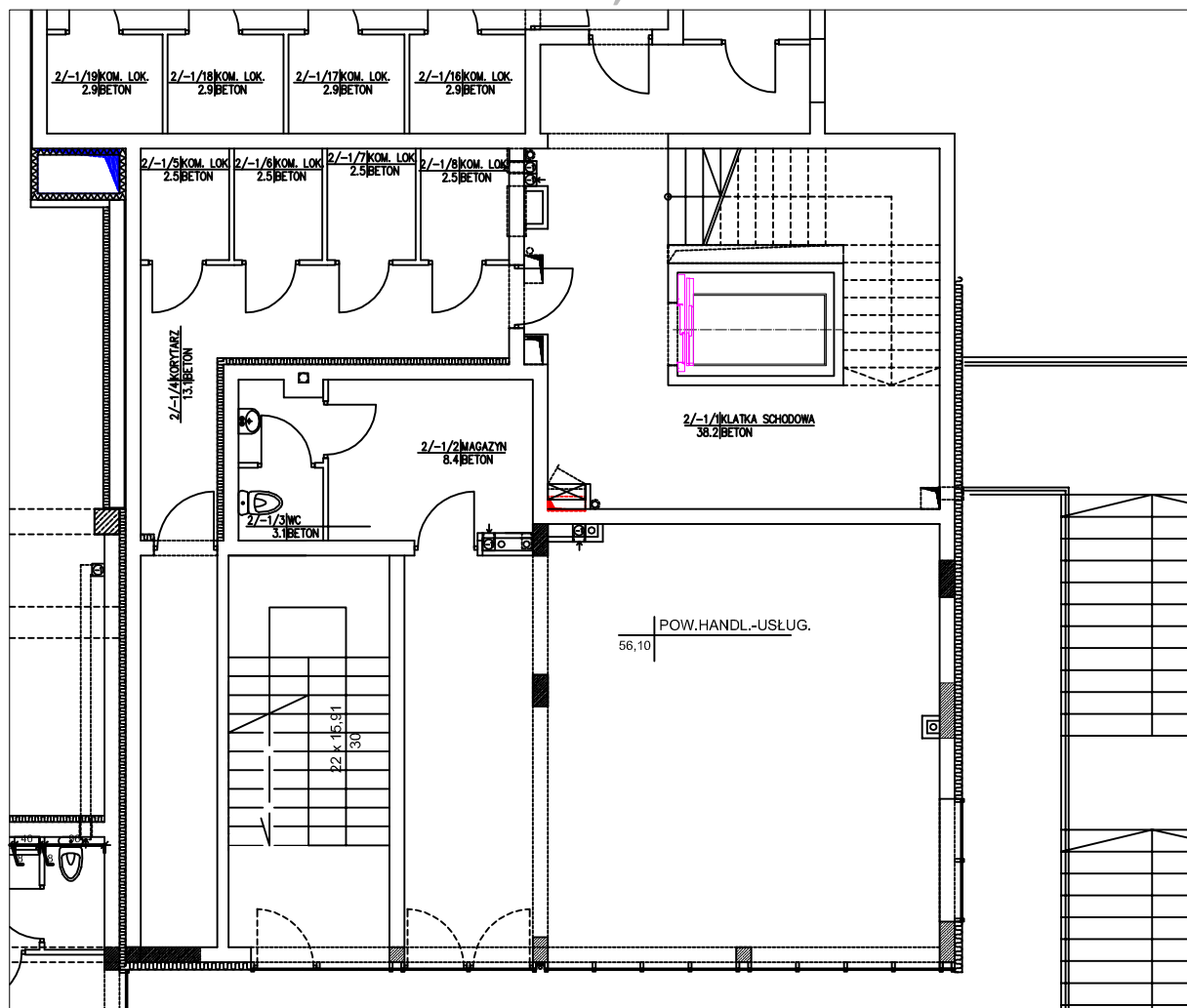
RZUT PARTERU:
